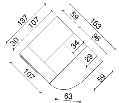
Grundriss rechter Schrank
